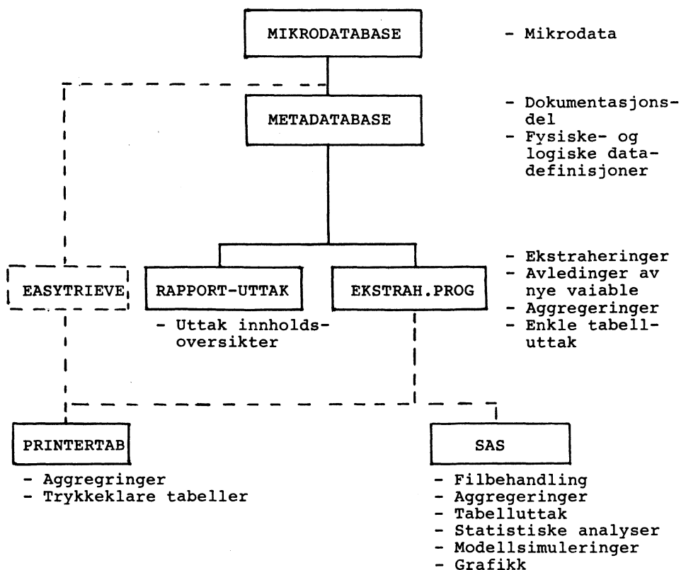
Figur 5.1. Oversikt over uttaksprogrammer i tilknytning til databasen
