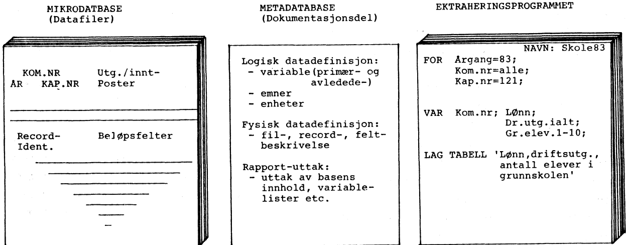
Figur 3.1. Databasens prinsipielle oppbygging. Eksempel på datastruktur i mikrodatabase, stikkordmessig beskrivelse av metadatabasen og eksempel på ekstraheringsprogram-spesifikasjoner ved et enkelt tabelluttak
