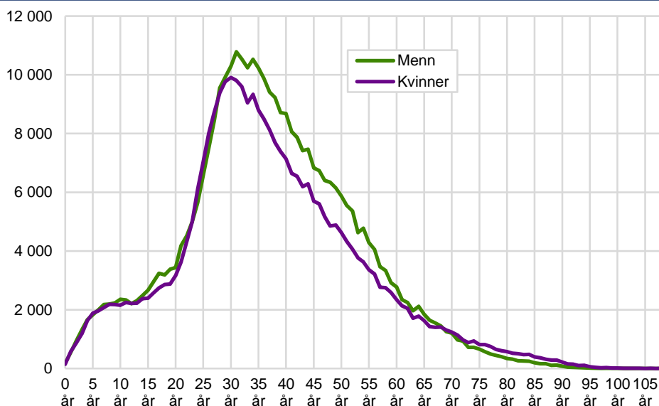
Figur 2.3. Innvandrere i Norge, etter kjønn og alder. 2015. Absolutte tall
