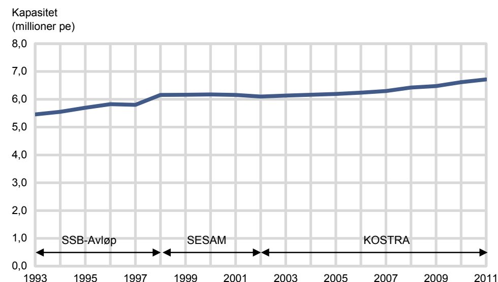
Figur 3.1. Kapasitet for avløpsanlegg dimensjonert for 50 pe eller mer. 1993 - 2011. Millioner pe
