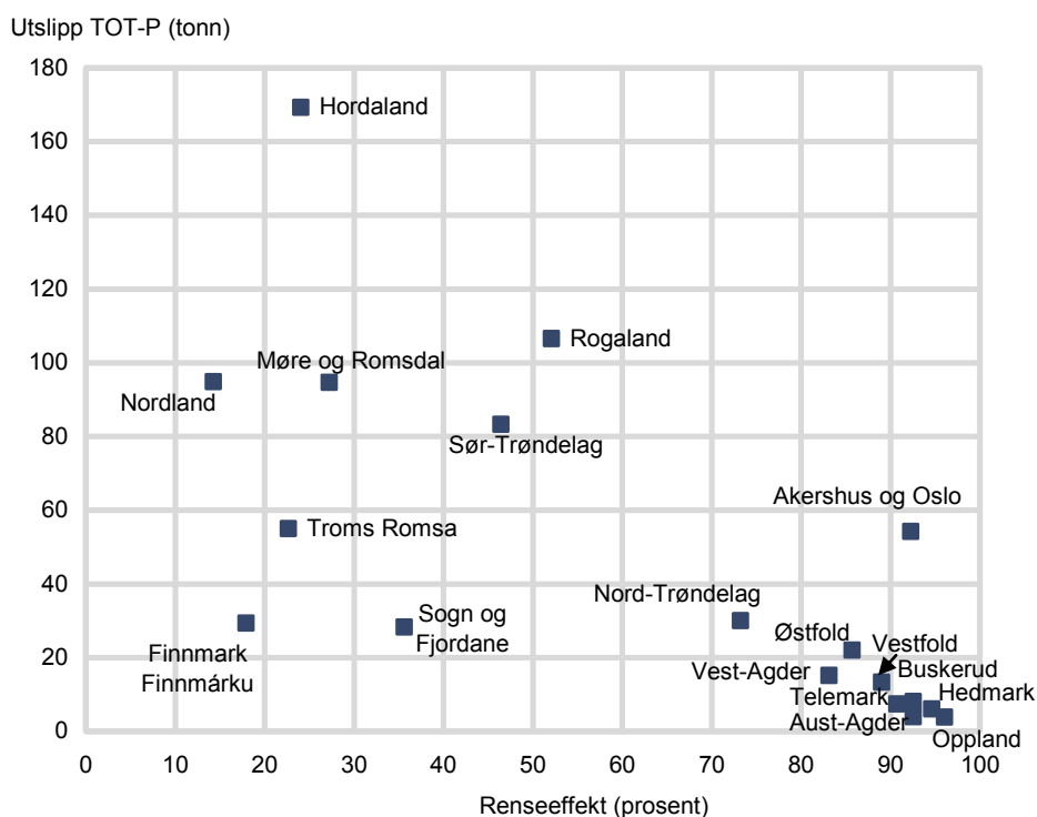
Figur 4.11. Utslipp og renseseffekt for fosfor i kommunal avløpssektor (anlegg ≥ 50 pe). 2011. Fylke
