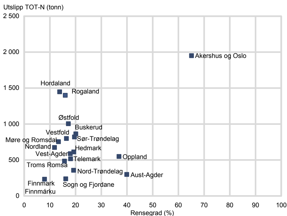
Figur 4.12. Utslipp og renseeffekt for nitrogen i kommunal avløpssektor (anlegg \geq 50 pe). 2011. Fylke
