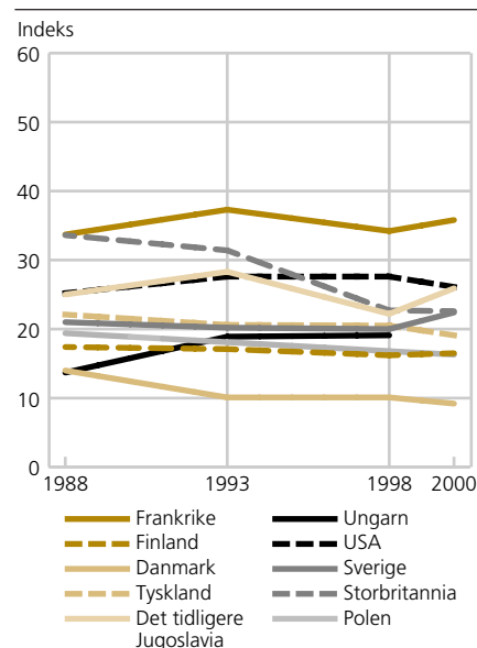
Figur 1. Dissimilaritetsindeks 1 for utvalgte vestlige og øst-europeiske innvandrergroper i Oslo, etter landbakgrunn og år. Antall poeng
