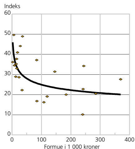
Figur 5. Dissimilaritetsindeks 1 og familieformue per forbruksenhet (gjennomsnitt) for utvalgte innvandrergupper bosatt i Oslo per 1.1.1998
