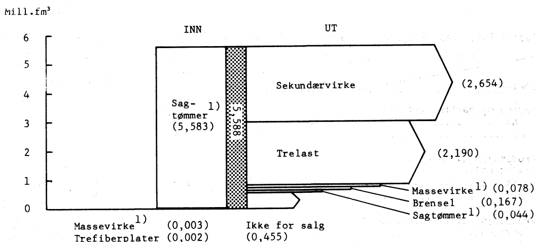
Figur 5.1 Strømningen av trevirke gjennom sektoren saging og høvling. 1981. 1 cm = 1 mill.fm 3
