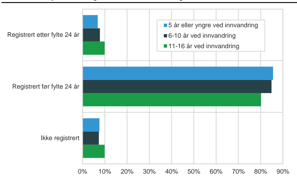
Figur 5.4 Andel med studiekompetanse fra videregående opplæring som har vært registrert i høyere utdanning, etter alder ved innvandring. Kvinner
