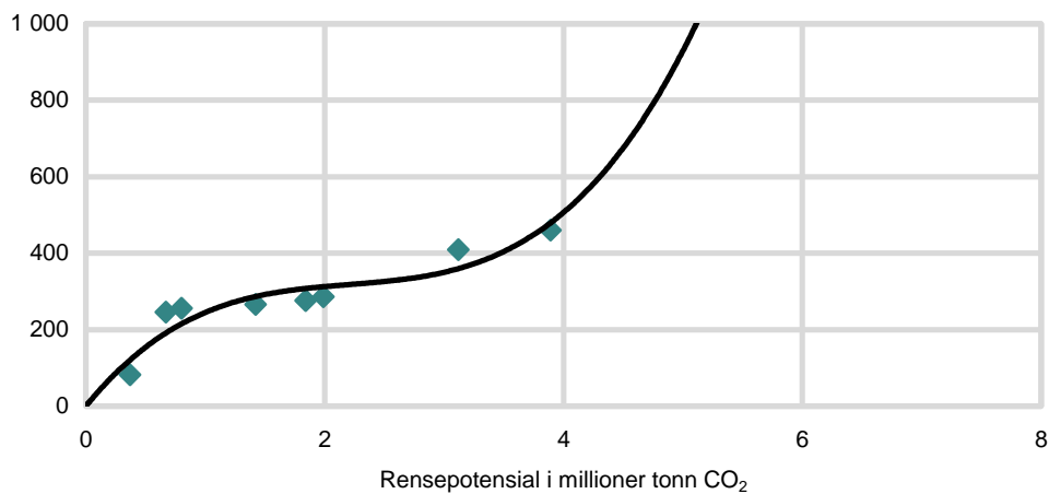
Figur A4. MSG-TECH: Marginale rensekostnadskurver for norsk petroleumsindustri. USD/tonn CO 2
